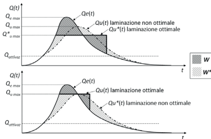
Figura 2 - Laminazione ottimale a parità di volume invasato W (sopra) e a parità di portata uscente massima Q_{u,max} (sotto)
